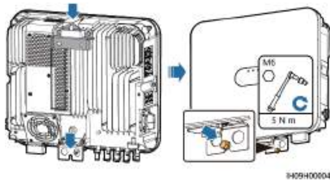
Figure 4-14 Serrage des boulons
