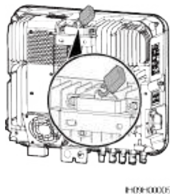
Figure 4-15 Installation d'un cadenas antivol
