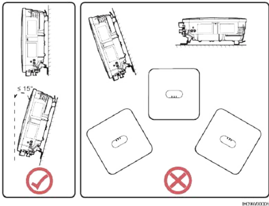
Figure 4-5 Angle d'installation
