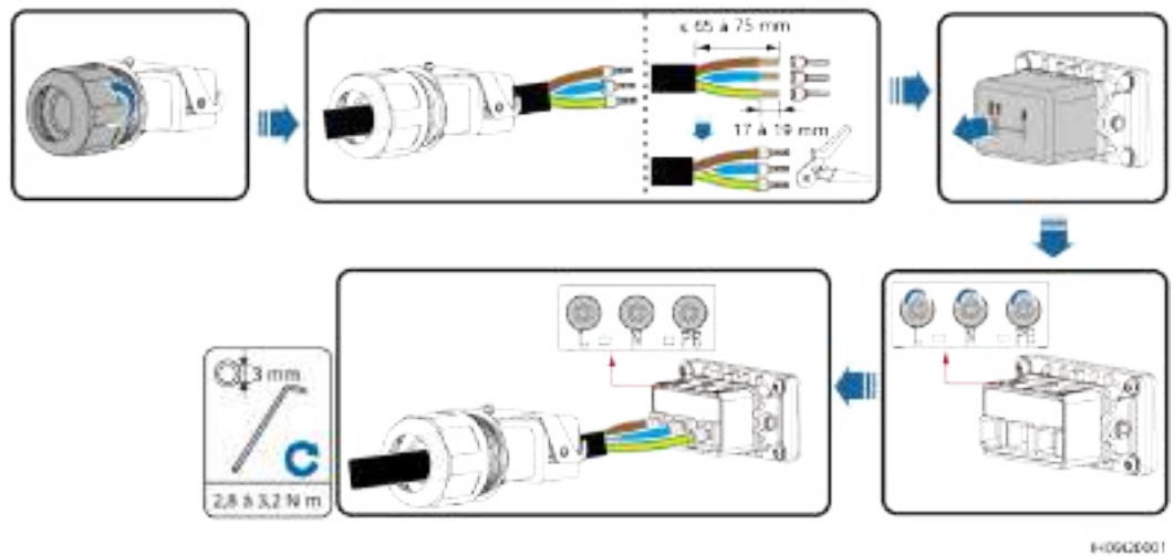
Figure 5-4 Installation du câble d'alimentation CA
