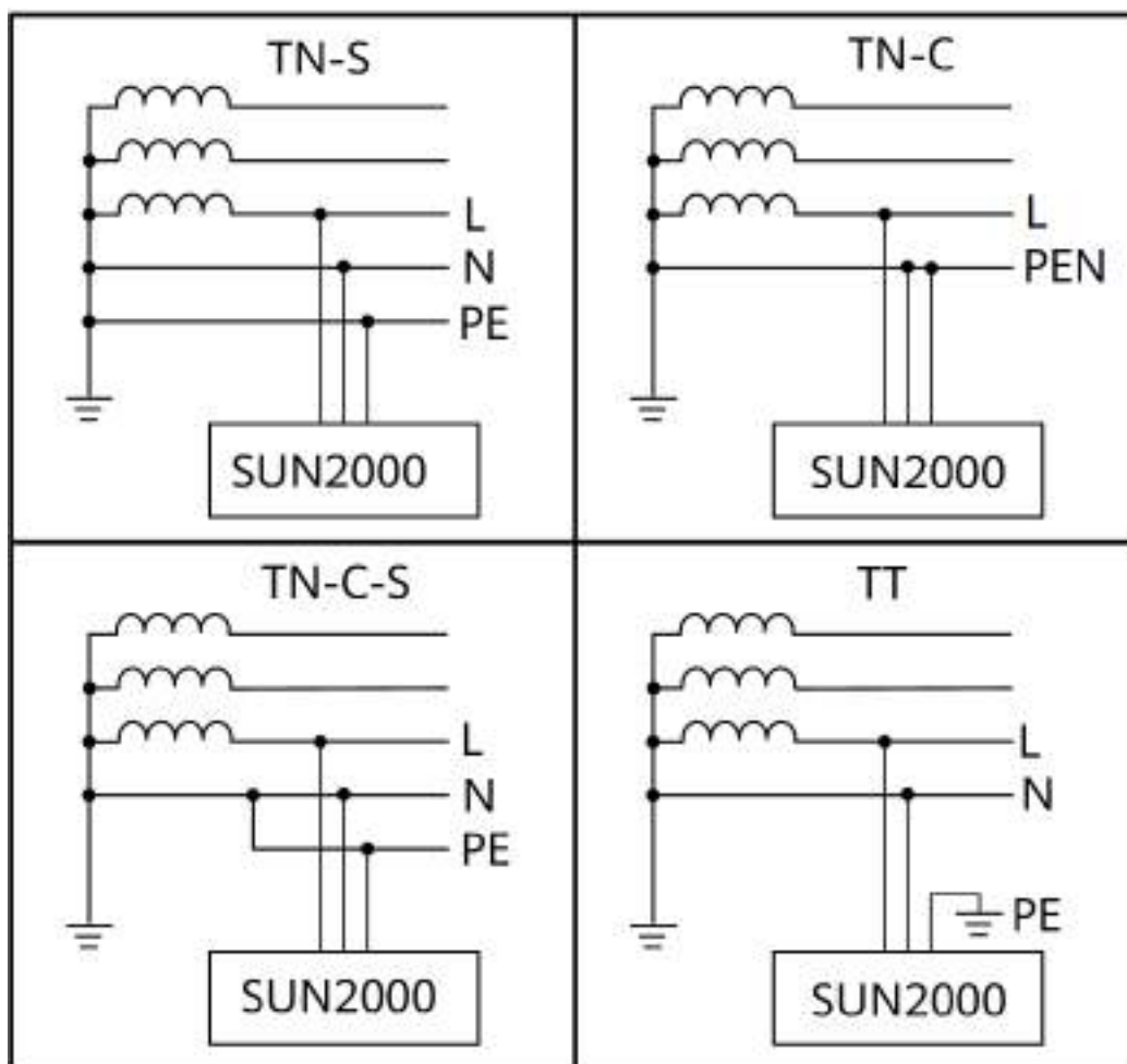
Figure 2-5 Types de réseau électrique
