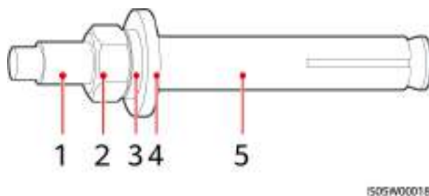
Figure 4-7 Composition d'un boulon à expansion
