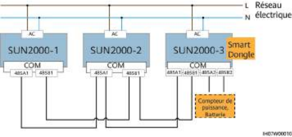
Figure 5-14 Mise en réseau du Smart Dongle (les composants dans l'encadré en pointillé sont facultatifs)
